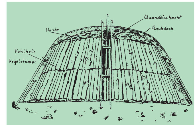
Querschnitt durch den Meiler
